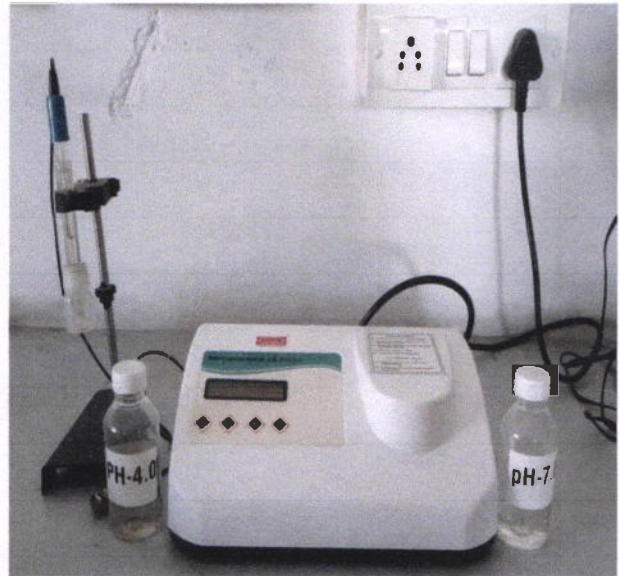
pH Meter
